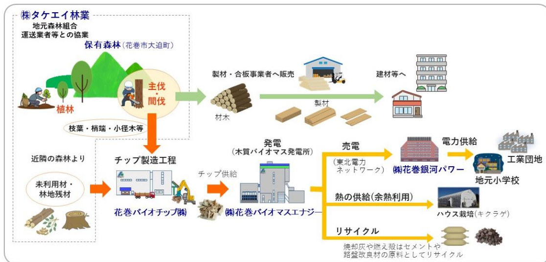
森林整備に基づく木質バイオマス発電事業のフロー図(花巻モデル)
